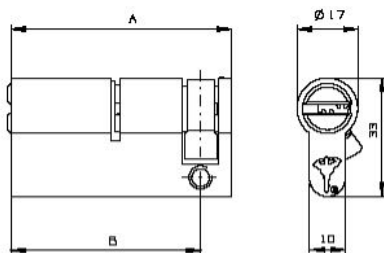
Рис.2. Габаритні розміри
