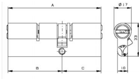
Рис.1. Габаритні розміри
